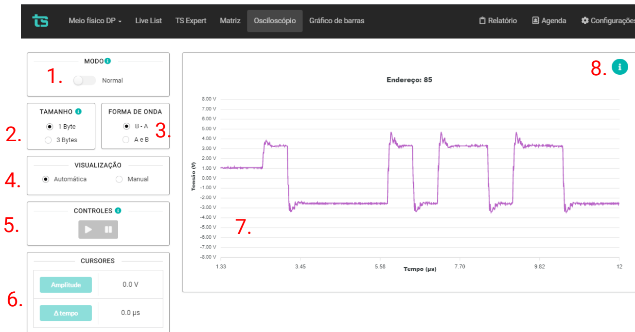
Figura 39: Tela Osciloscópio (B - A)
