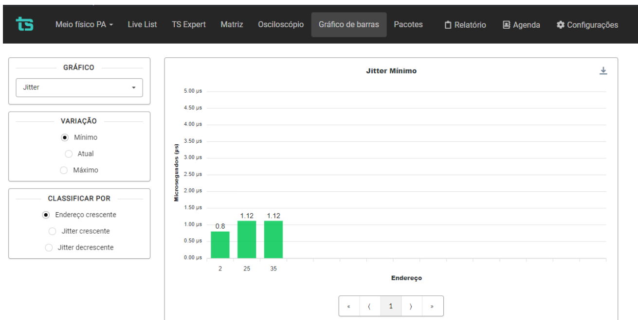
Figura 58: Tela Gráfico de barras (Jitter)
