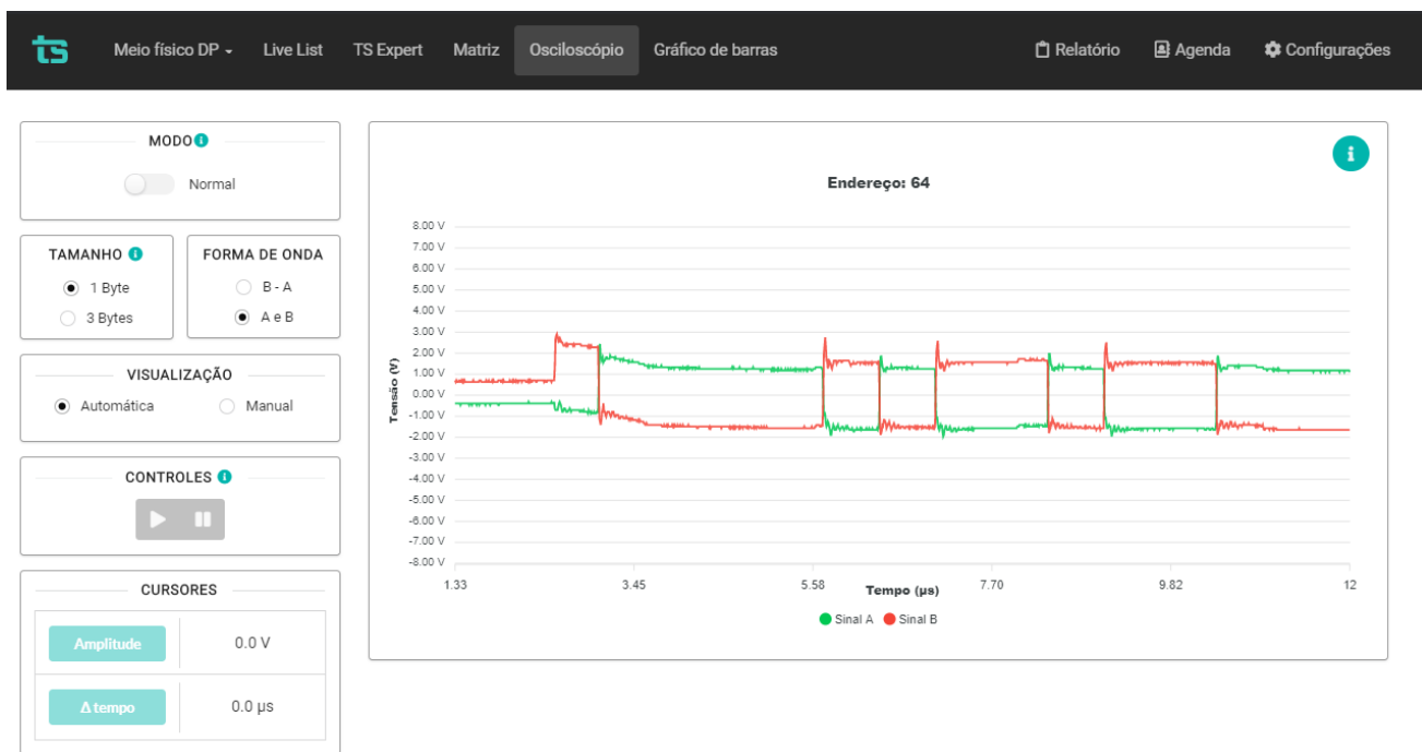
Figura 40: Tela Osciloscópio (Sinal A e B)
